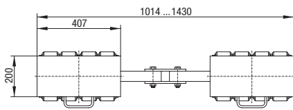
Typ / Model F18
