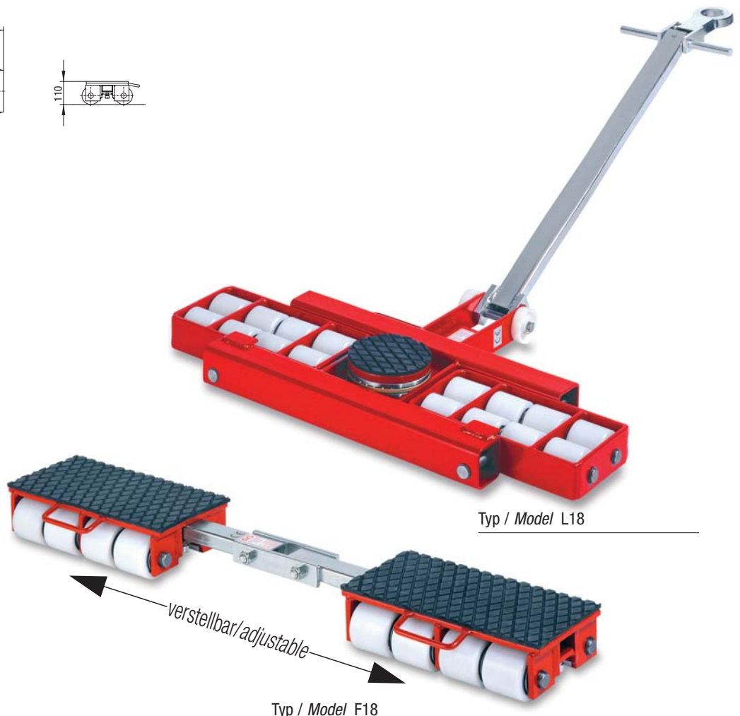
Typ / Model L18, lenkbar / steerable
