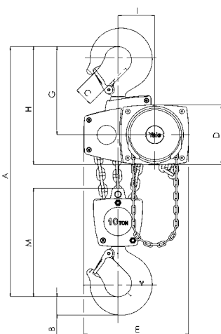
Modell Yalelift 360, 10.000 kg, dreisträngig
